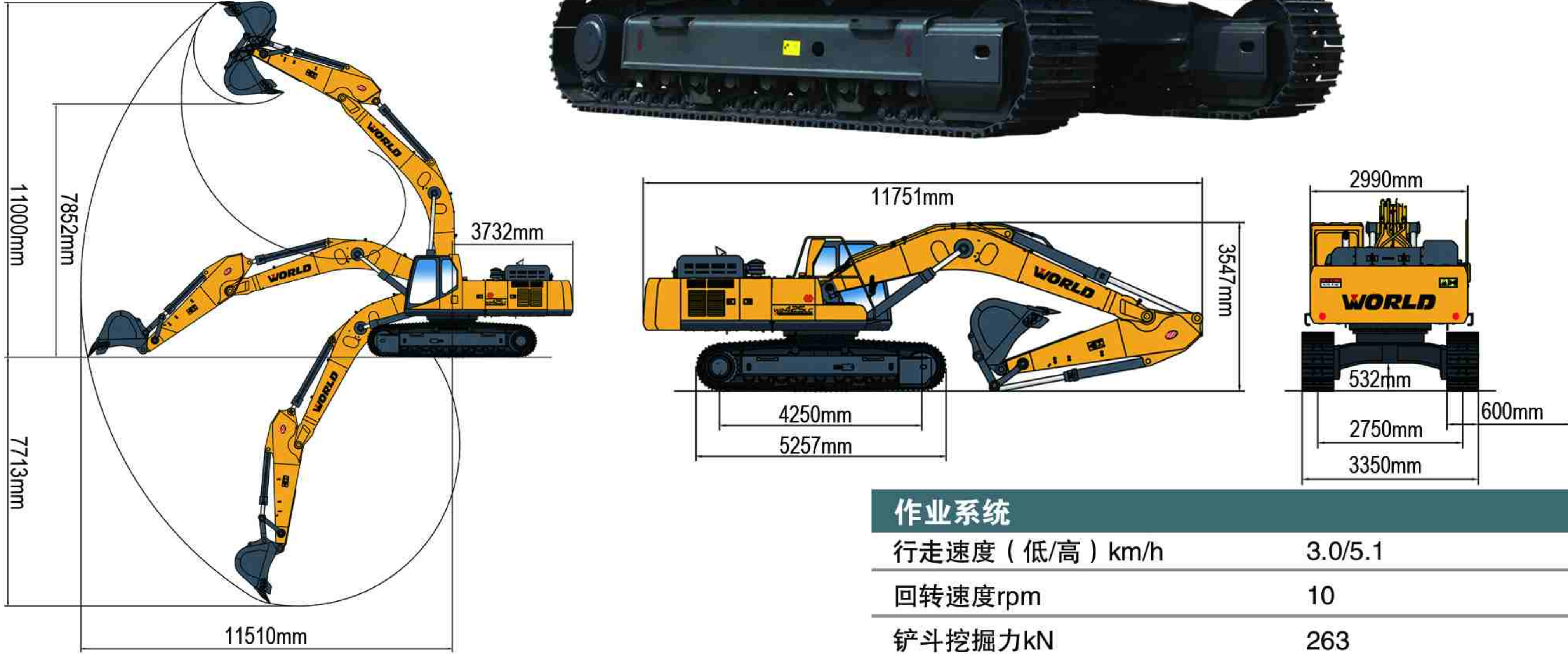
W2425LC-8尺寸图
